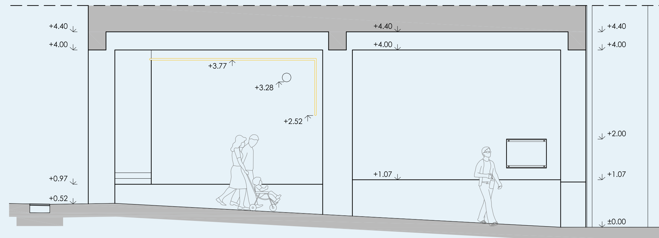
S01-S01
