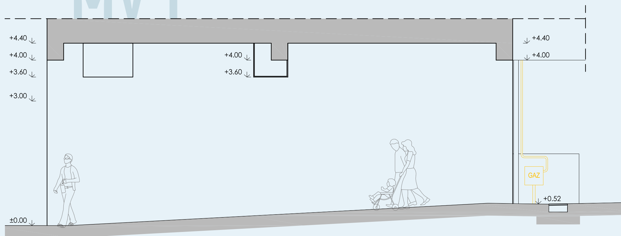
S02 - S02
