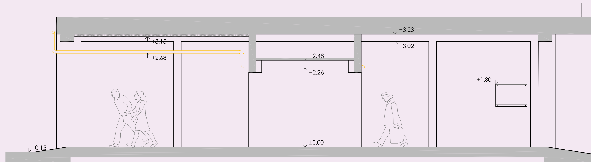
S01 - S01
