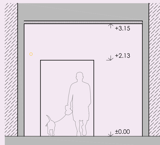
S04 - S04
